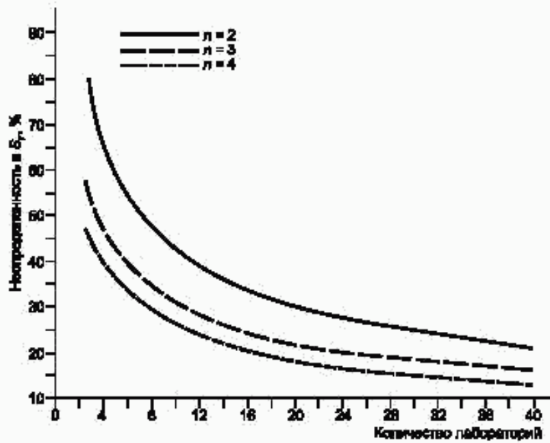
Рисунок В.1 — Ожидаемая величина, на которую s_p может отличаться от истинного значения на уровне вероятности 95 %
